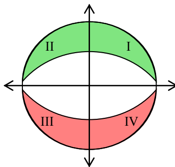
sine
