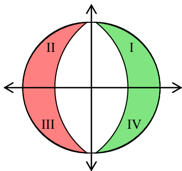
cosine
